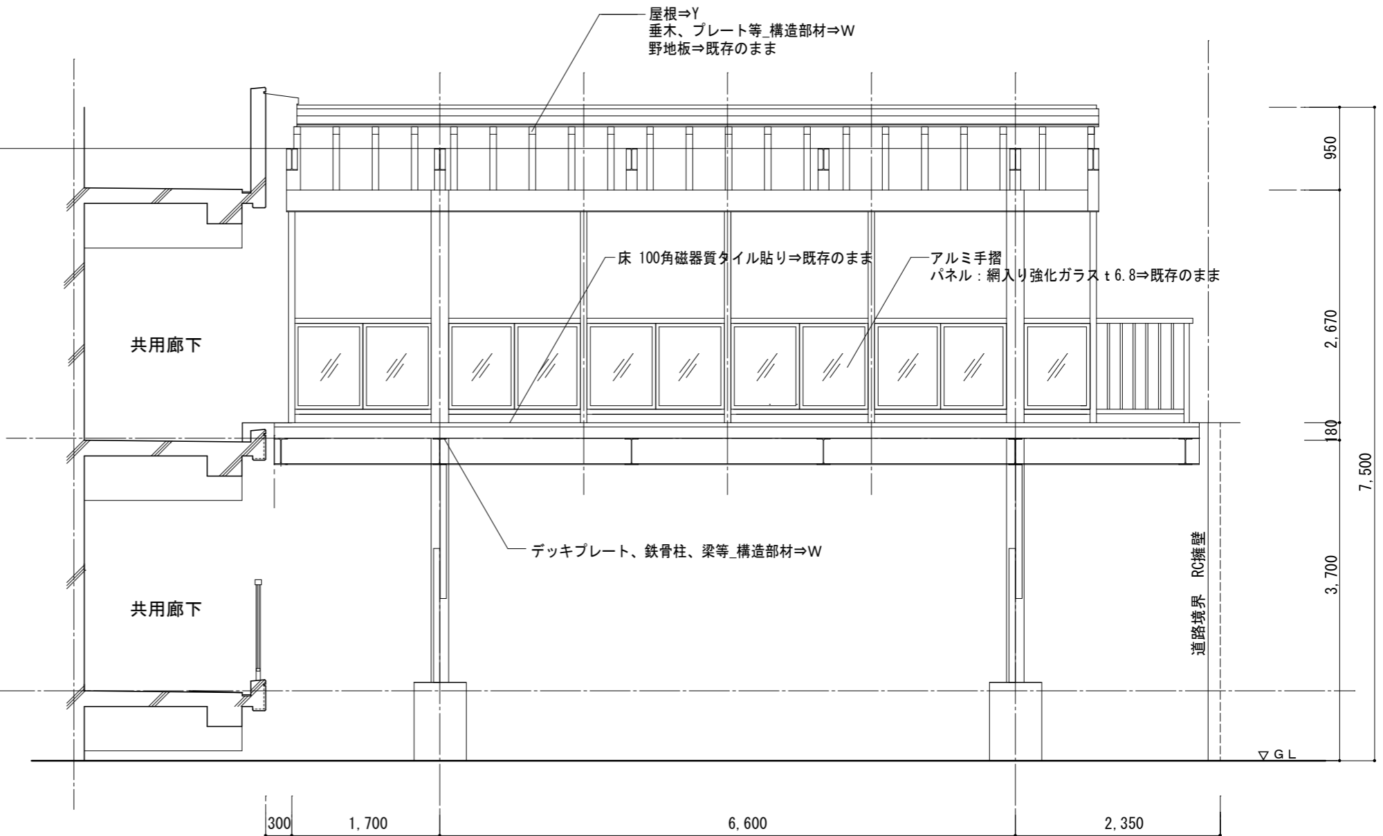
渡り廊下 矩形図
