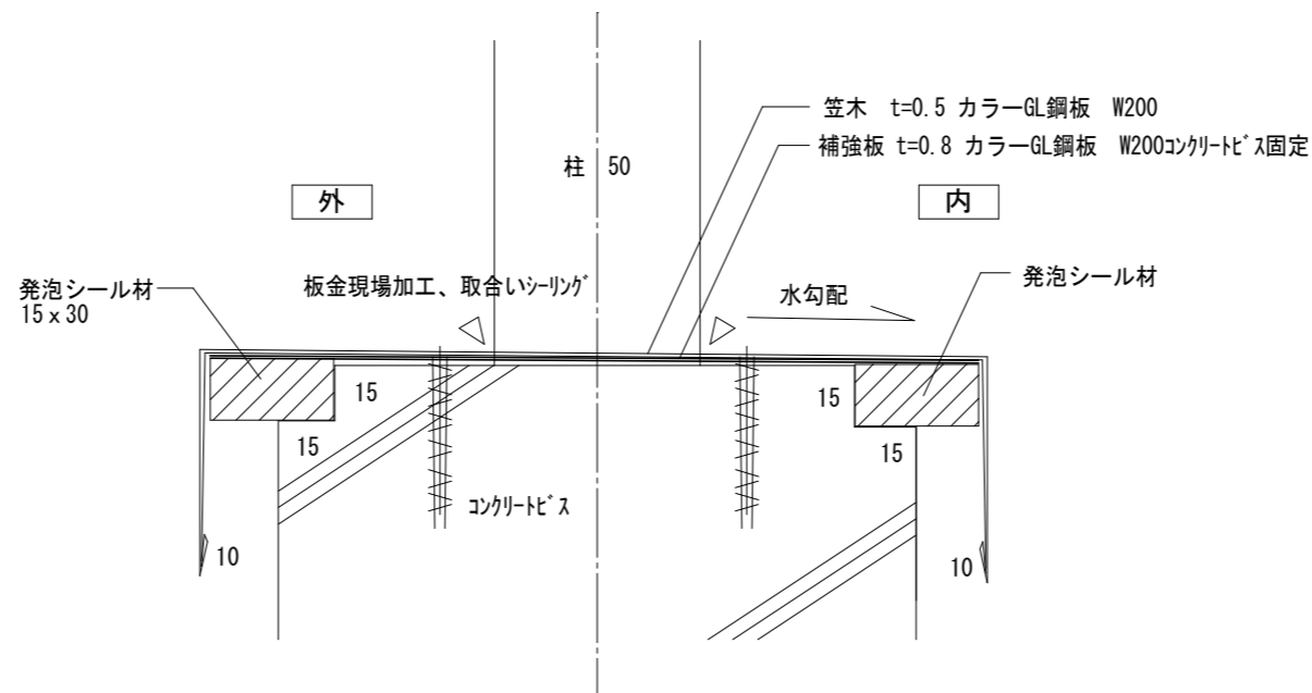
バルコニー手摺下部笠木詳細図
