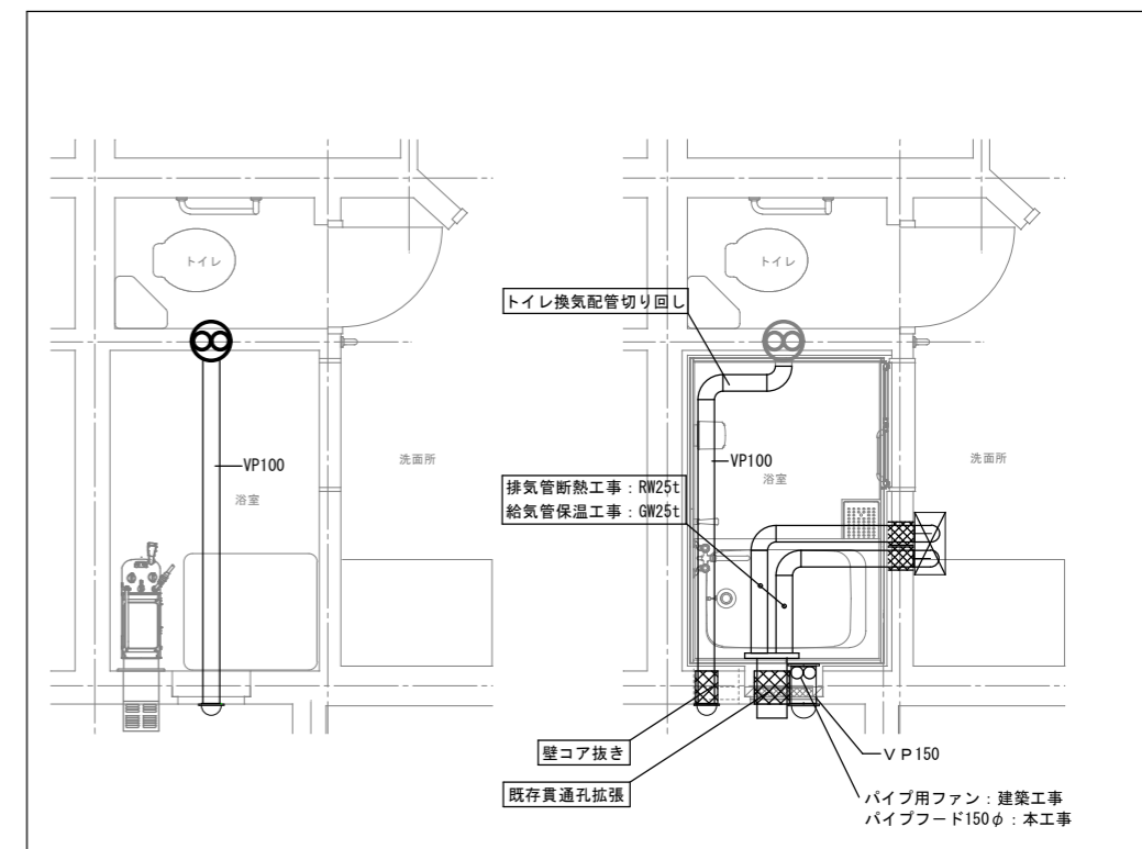
改修前 平面詳細図 (換気) S=1:25
