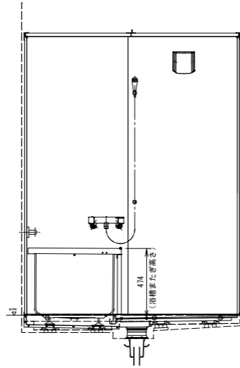
[在来工法床面設置の場合 (MR工法)]
