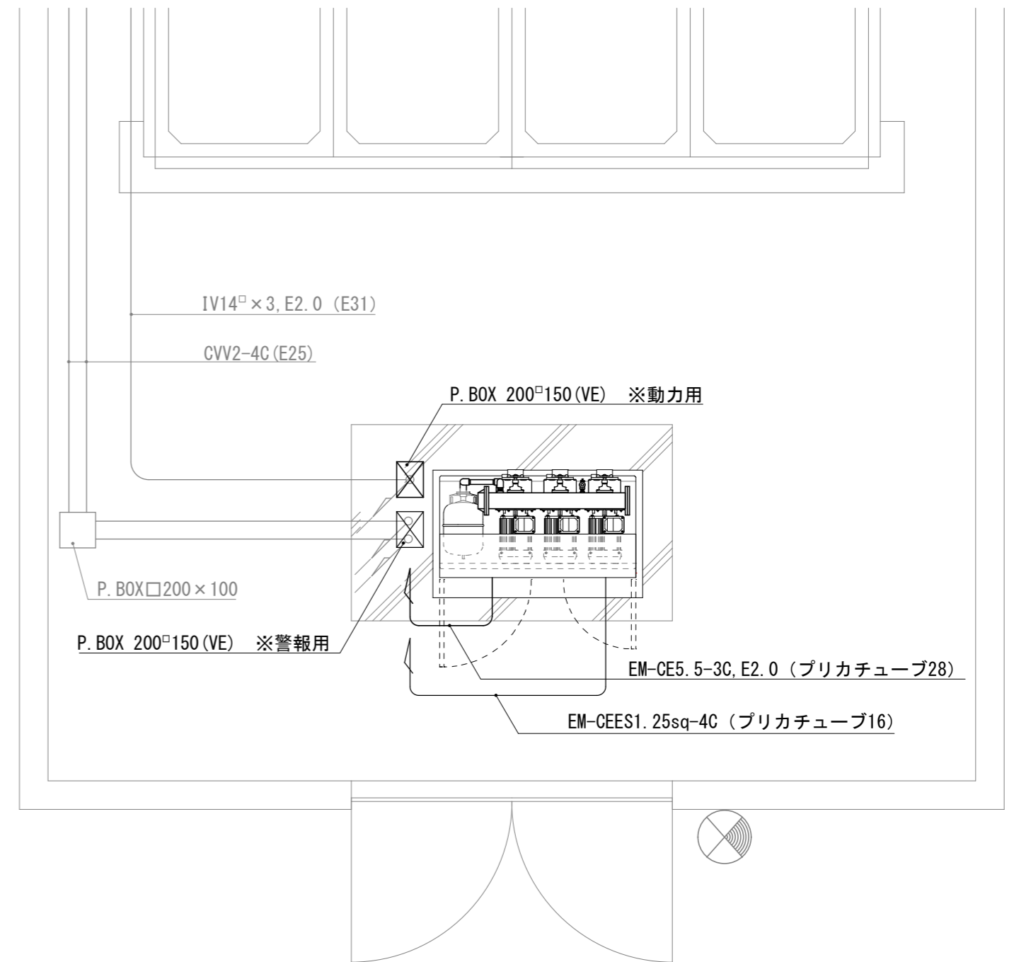
改修平面図
