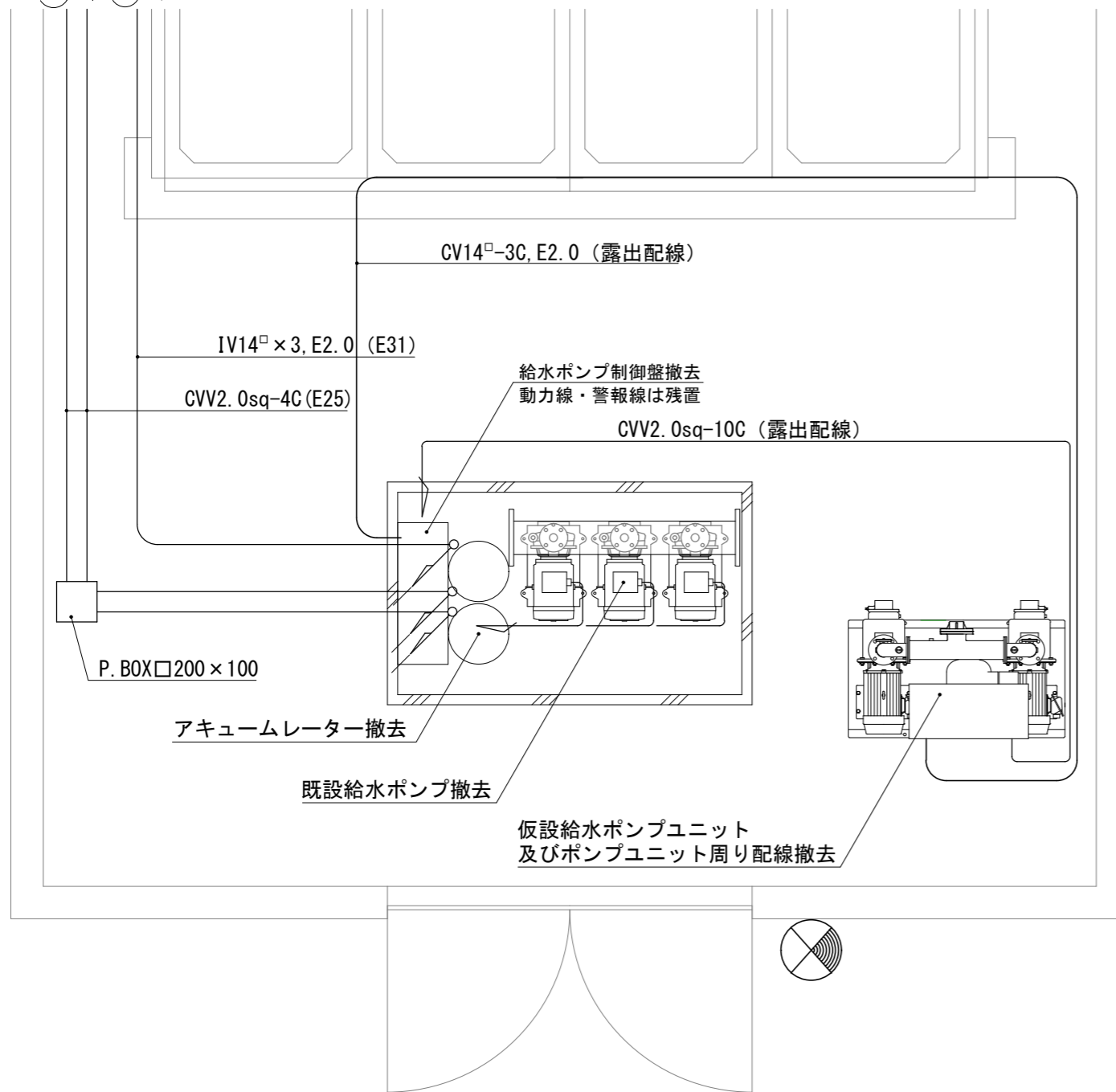
既存平面図
