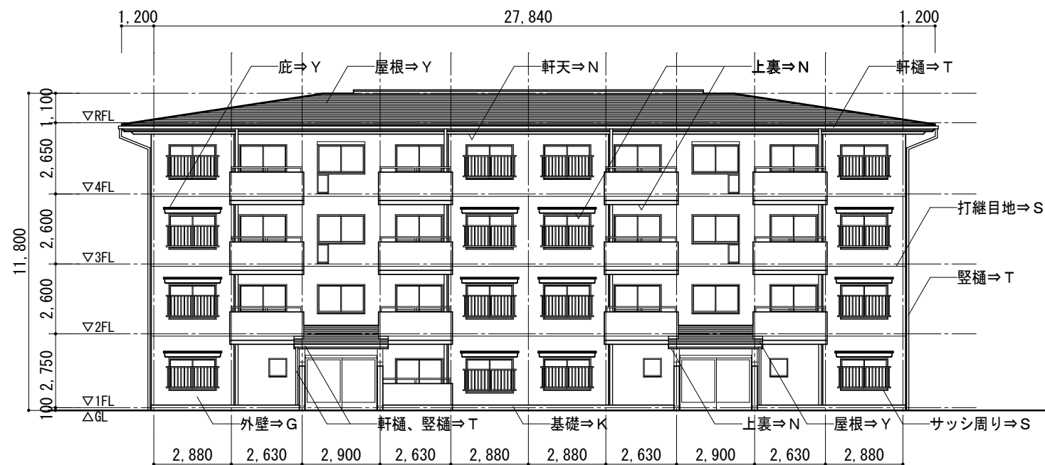
北立面図 S=1/200
