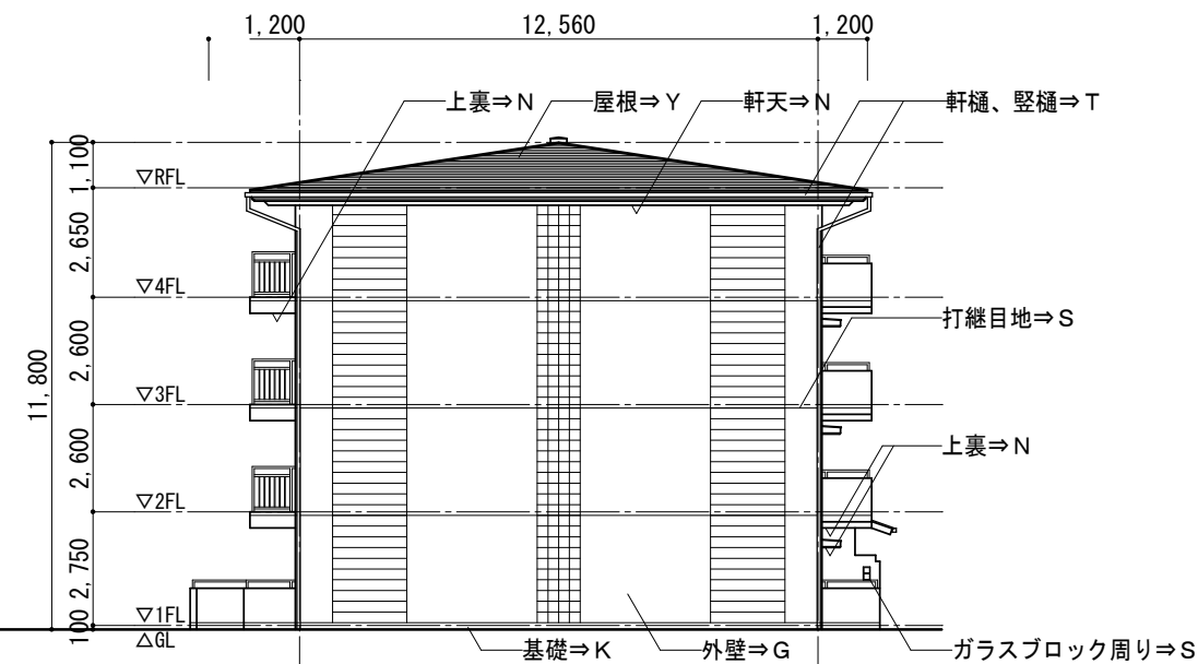
東立面図 S=1/200
