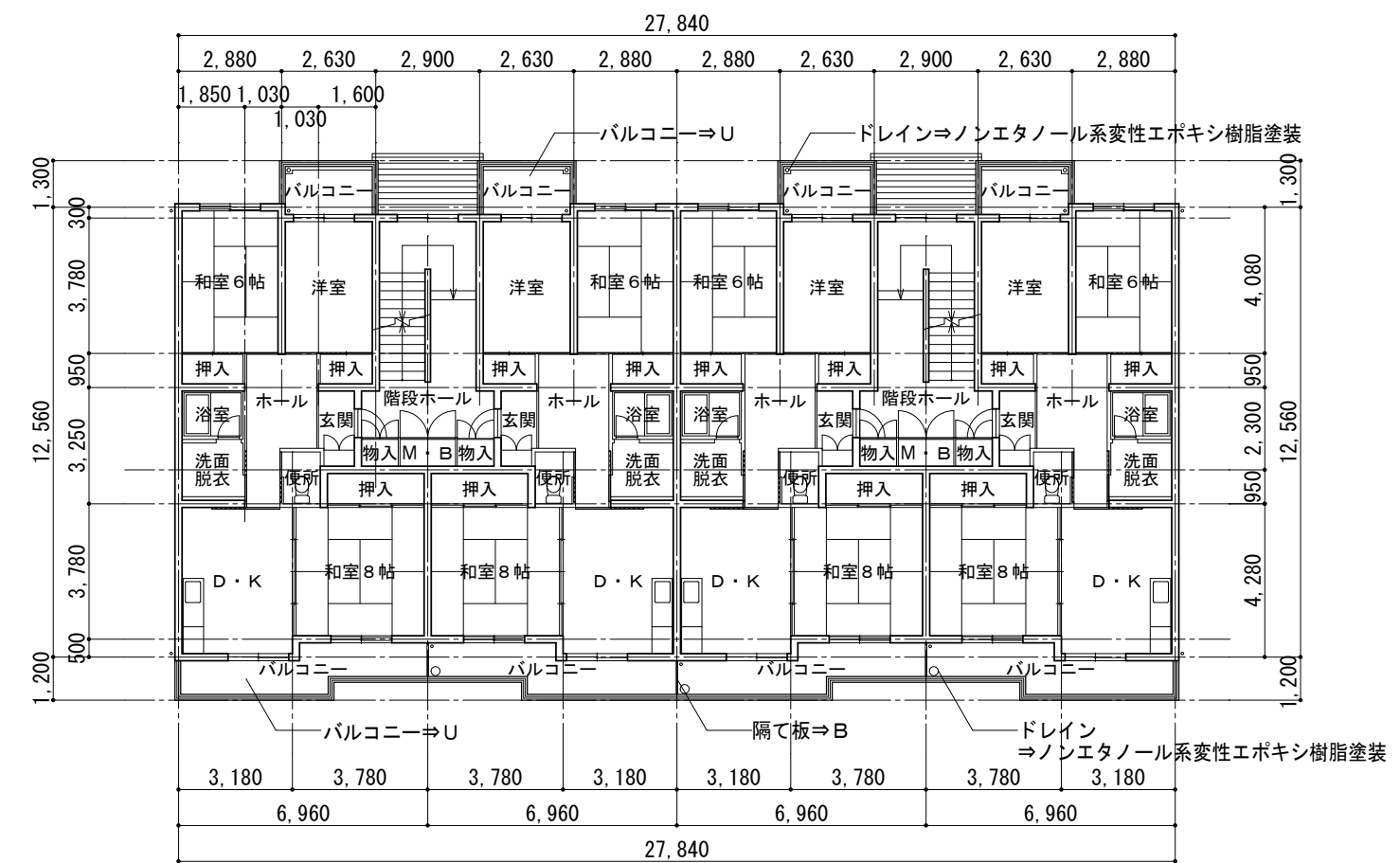
2～4階平面図 S=1/200
