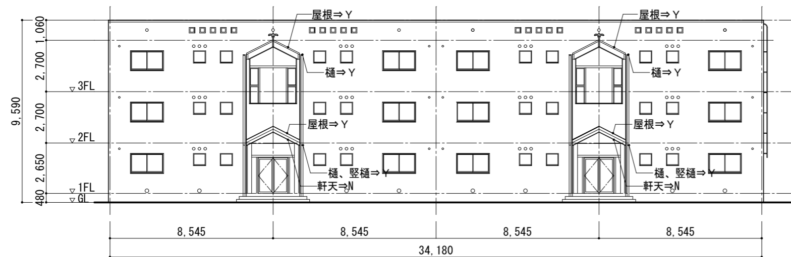
北立面図 S=1/200
