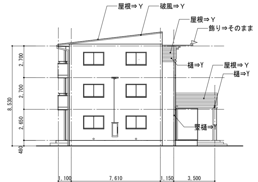
東立面図 S=1/200
