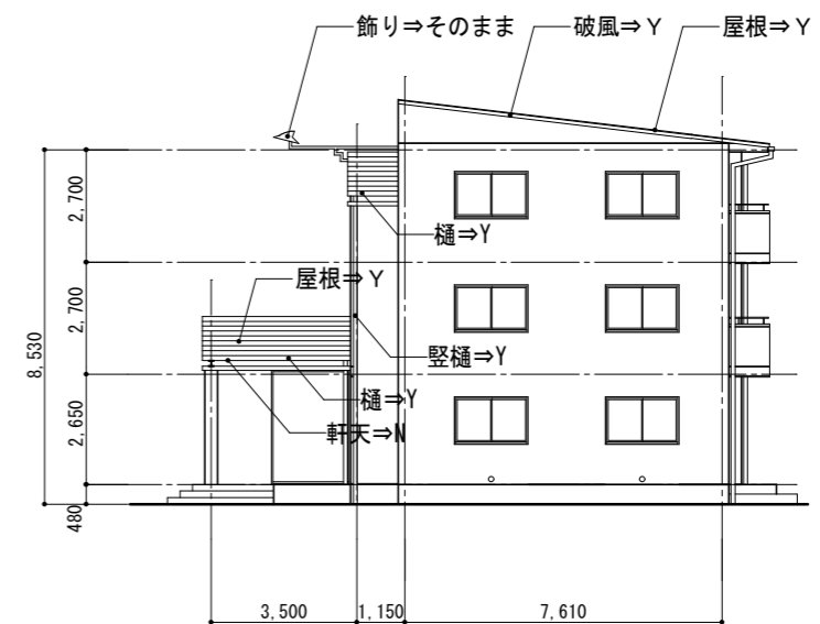
西立面図 S=1/200
