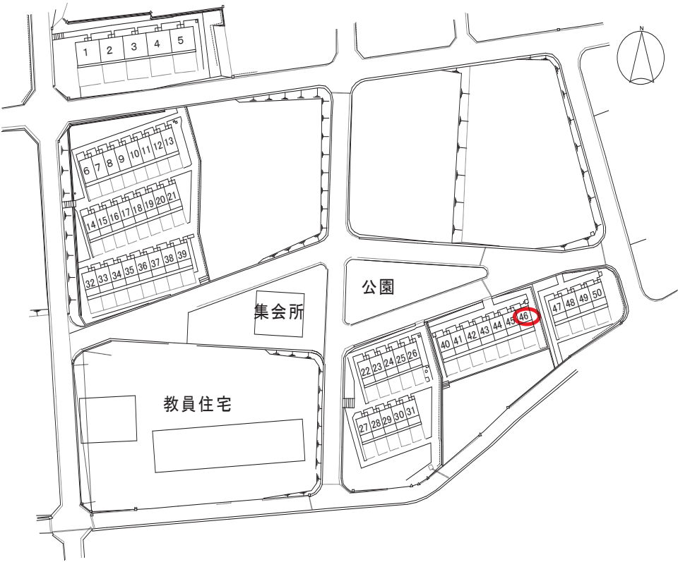
配置図
